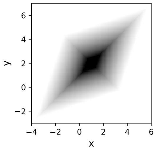
GeneralSersic2D, c=-1.0
