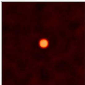
TrapezoidDisk2DKernel
