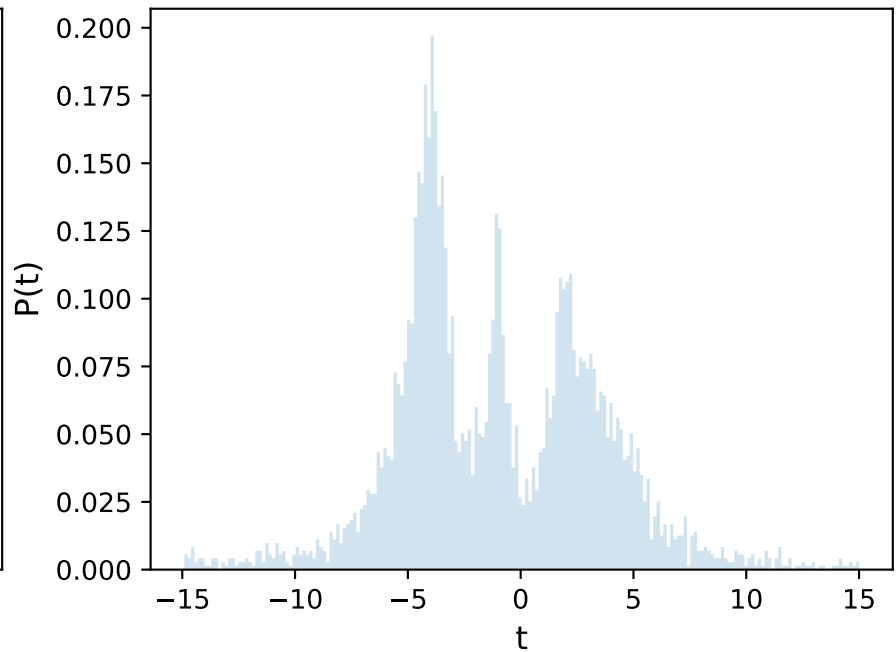
plt.hist(t, bins=200)
